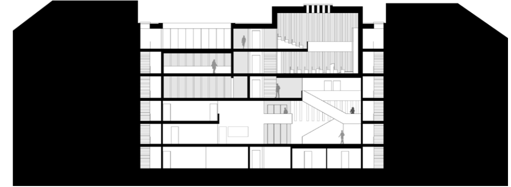
unten: Längsschnitt
