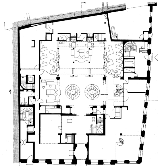
unten: Grundriss Erdgeschoss
